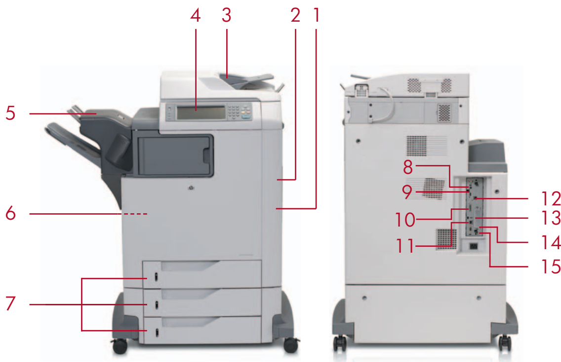
Urządzenie wielofunkcyjne HP Color LaserJet 4730xs mfp -widok z przodu
